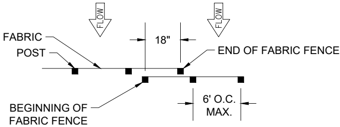
TOP VIEW N.T.S.
