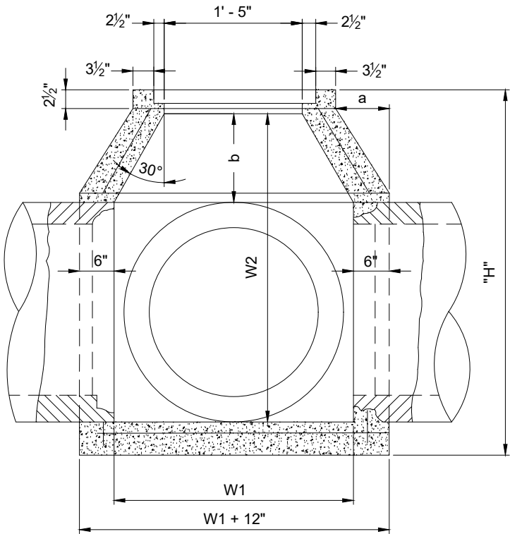
SECTION A-A
