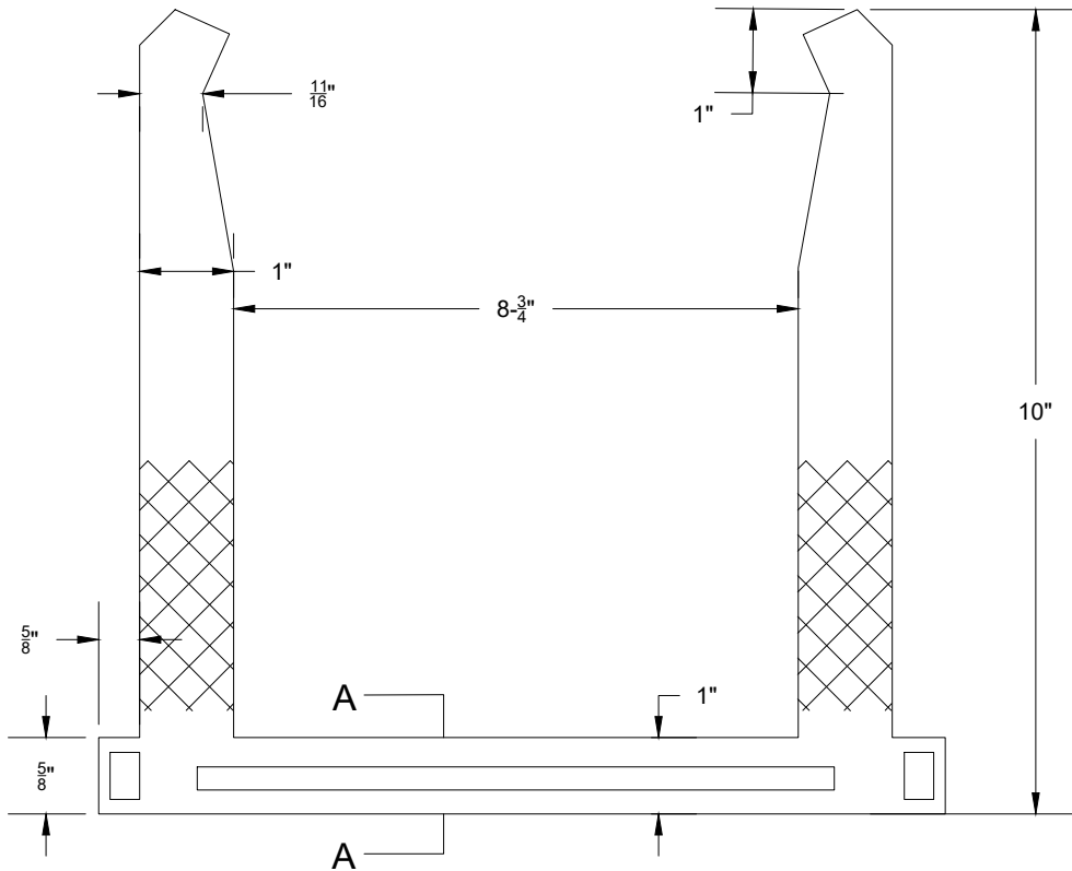
PLAN VIEW N.T.S
