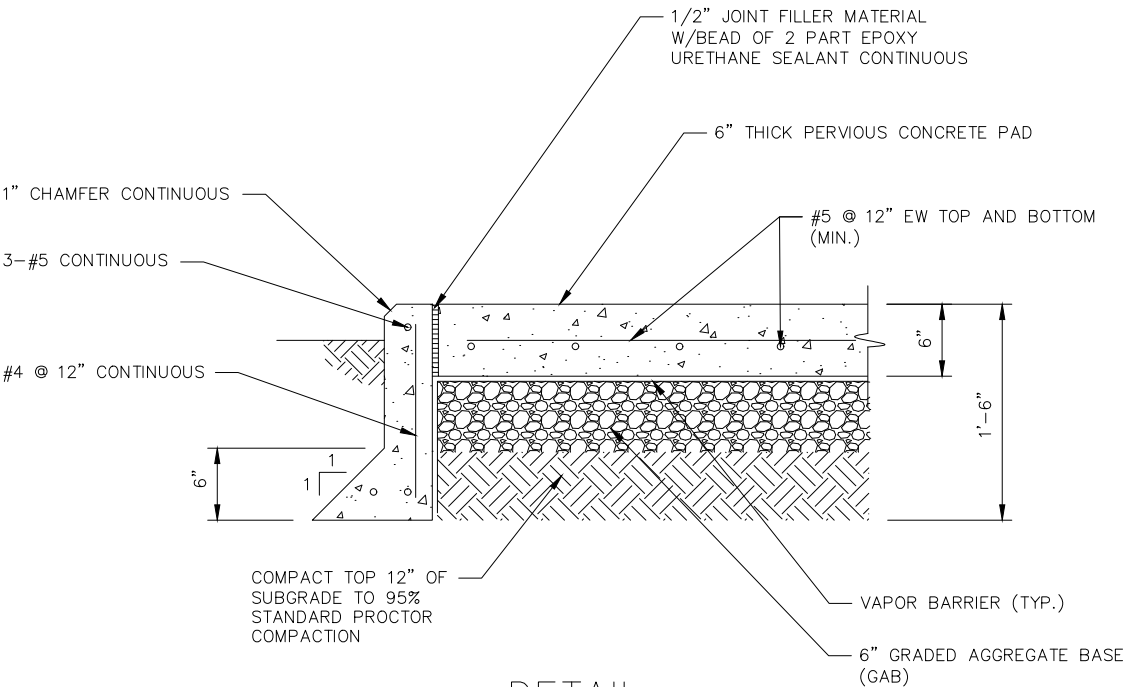
DETAIL N.T.S.
