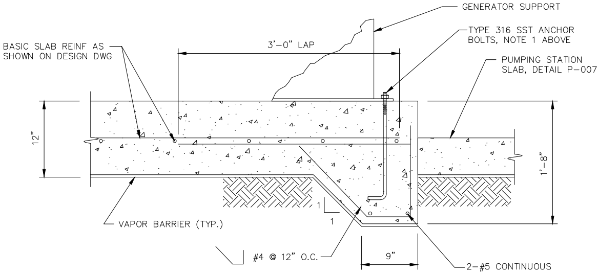
SECTION (TYP.) N.T.S.
