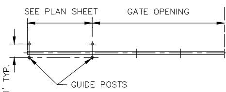
PLAN VIEW N.T.S.
