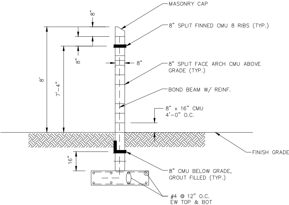
SECTION VIEW N.T.S.
