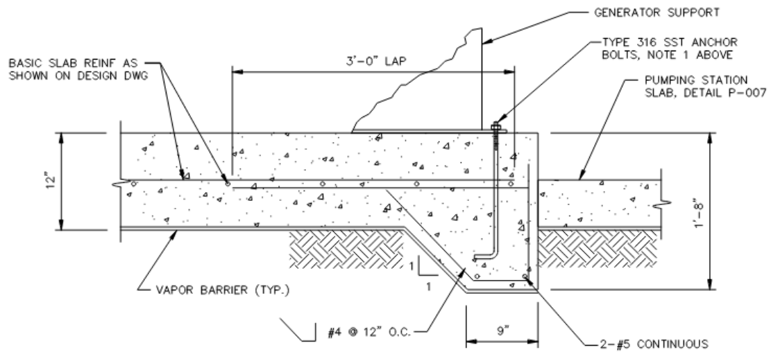
PLAN N.T.S.
